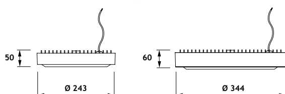
Mini - BY020P - Dimensions en mm
